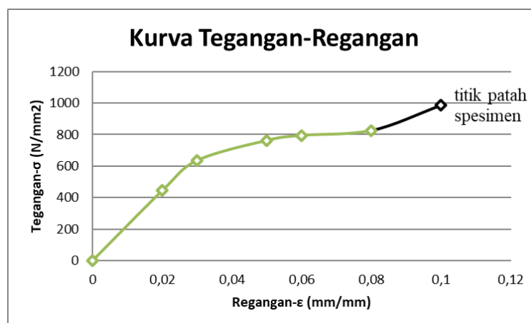
Gambar 2. Kurva Tegangan-Regangan
